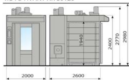
ROTO AVANT HR 80120
